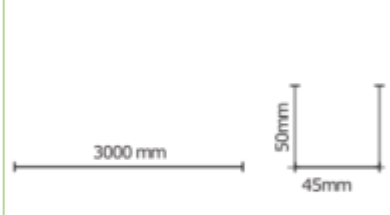
PROFIL CW 50
